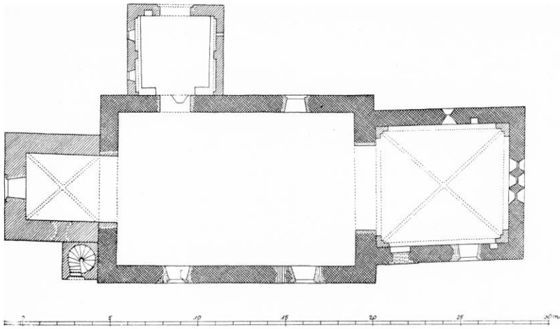
Fig. 2. Gundslev. Plan. 1:300. Målt af Aa. RI. 1940.
