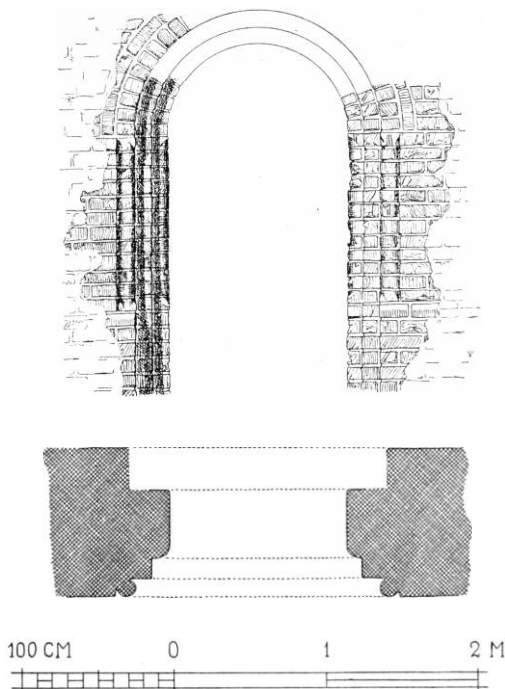
Fig. 3. Gundslev. Sydportal. 1:50. Målt af Aa. Rl. 1940 (s. 1160).
