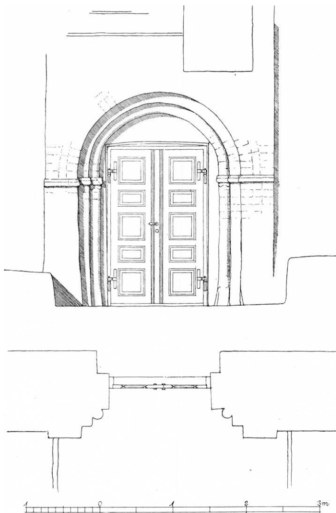
Fig. 4. Bregninge. Sydportal. 1:50. Målt af J. Heindorff 1944 (s. 1102).
