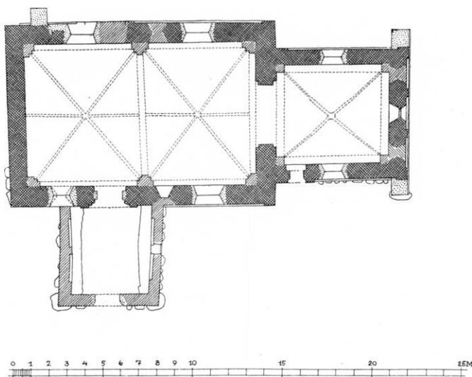
Fig. 2. Bregninge. Plan. 1:300. Målt af Aa. Rl. 1952.
