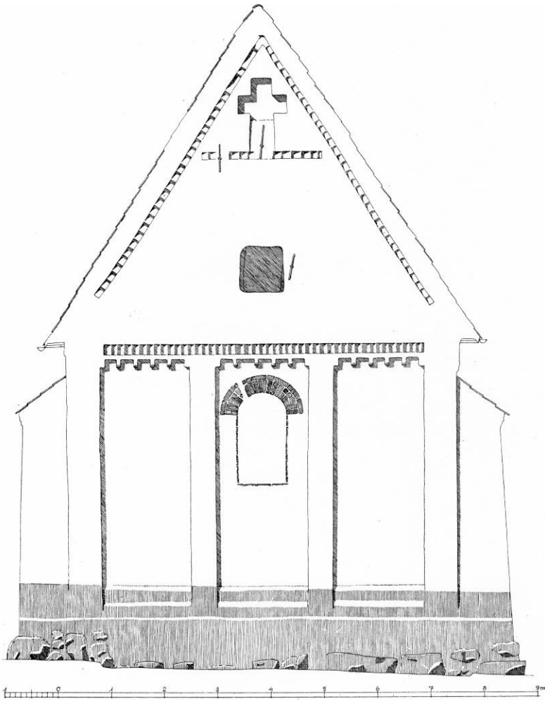
Fig. 3. Bregninge. Østgavl. 1:100. Målt af H.A.Poulsen 1944 (s. 1102).
