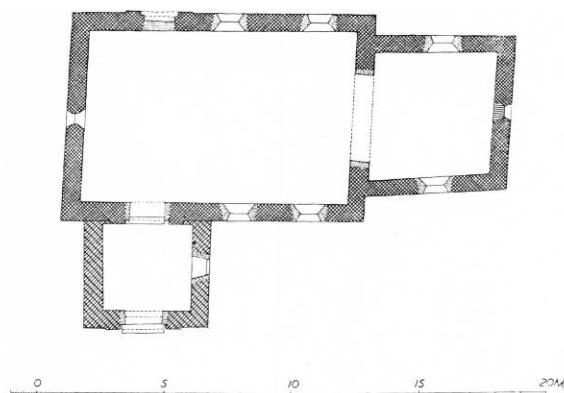
Fig. 2. Krønge. Plan. 1:300. Målt af Grethe Meyer 1944.
