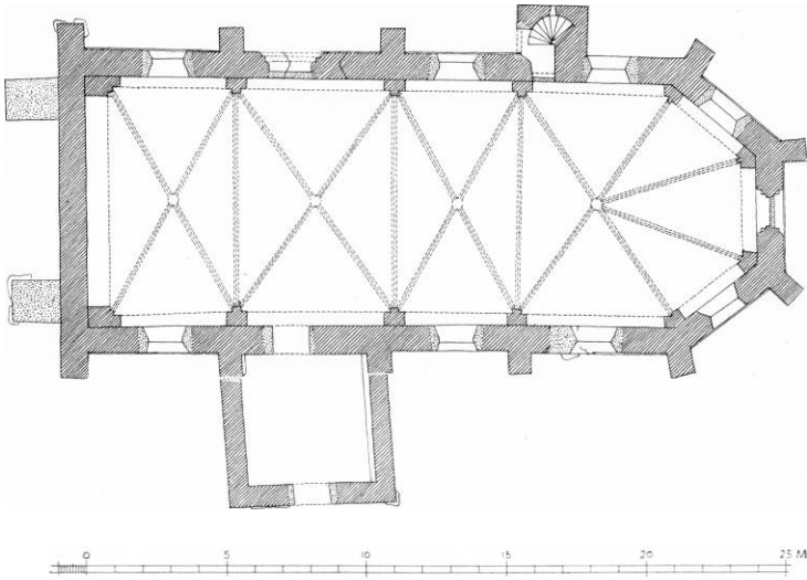
Fig. 2. Vesterborg. Plan. 1:300. Målt af El. M. 1948.
