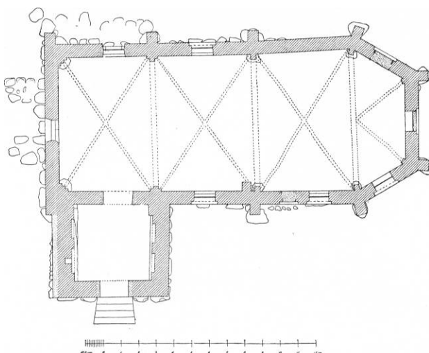
Fig. 2. Avnede. Plan. 1:300. Målt af Jens Sørensen 1942.
