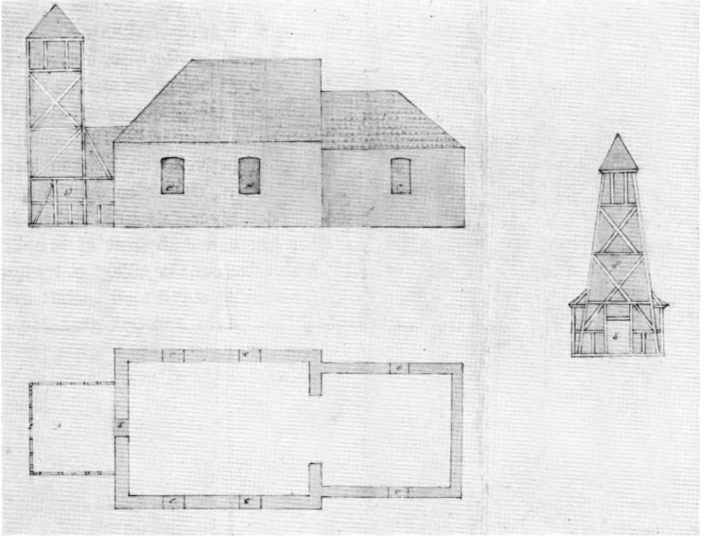
Fig. 1. Aageby. Plan, sydside og snit af klokketårn. 1:300. Opmåling af H. Erichsen, Stokkemærke o. 1775.
