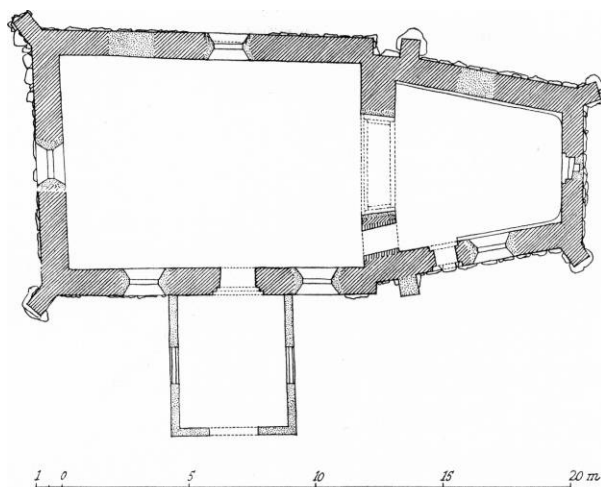
Fig. 2. Kappel. Plan. 1:300. Målt af Elna Møller 1948.
