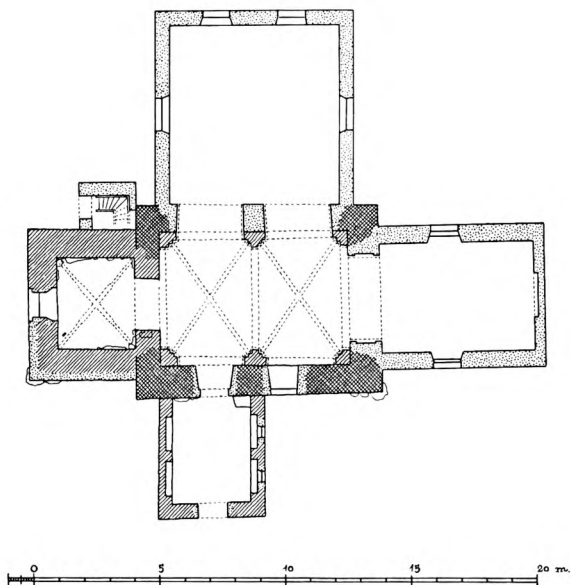
Fig. 2. Slagslunde. Plan. 1:300. Målt af C. G. Schultz 1935. Tegnet af Henrik Jacobsen 1975.
