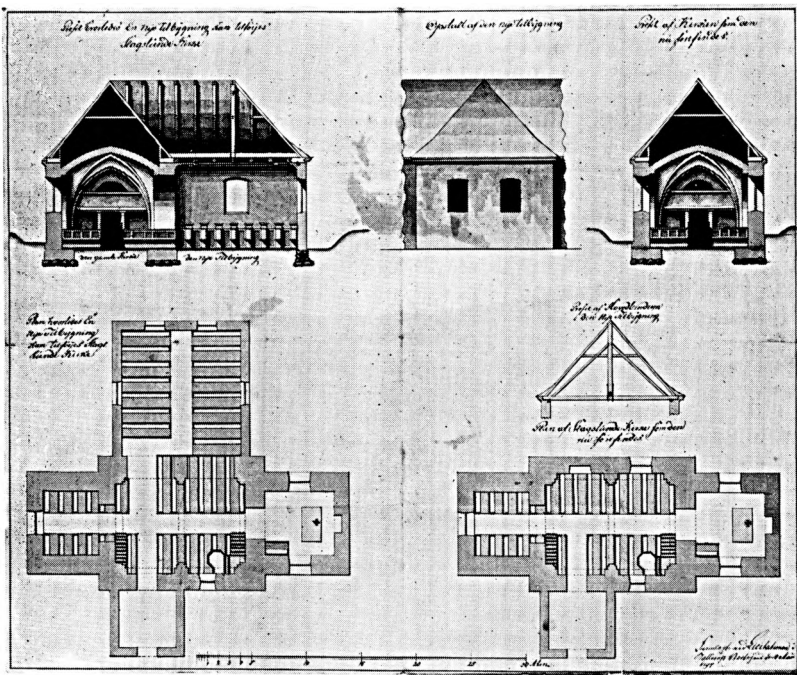
Fig. 3. Slagssunde. Hofbygmester, Johan Boye Junge Magens' 1797 approberede tegninger til den året efter opførte tilbygning. 1:450. Rigsarkivet.
