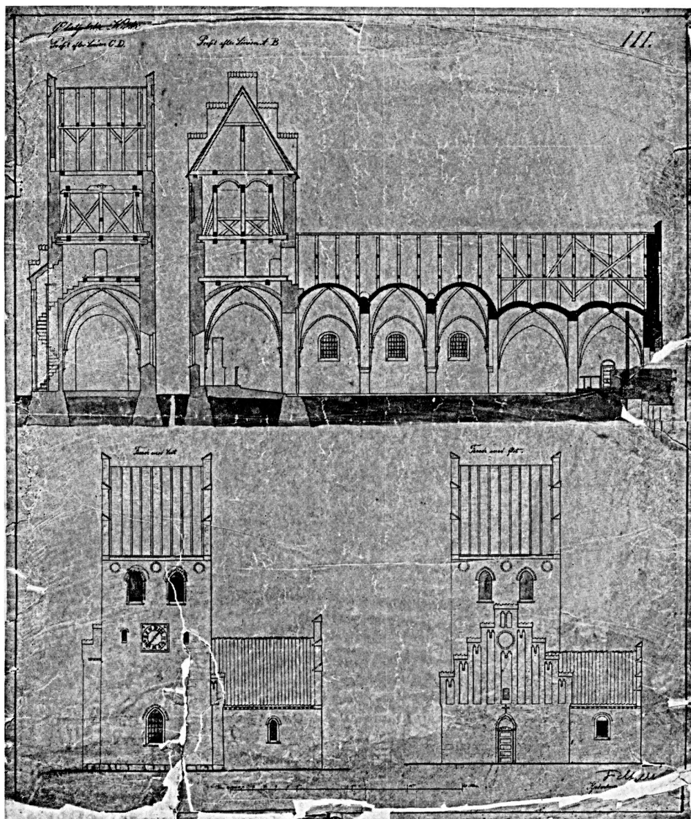
Fig. 4. Ølstykke. Tegning (i Rigsarkivet) af F. Meldahl til kirkens ombygning 1867.
