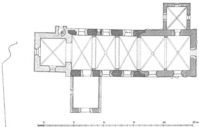
Fig. 2. Ølstykke. Plan. 1:300. Målt og tegnet af C. G. Schultz 1935 med enkelte suppleringer ved Hans Stiesdal 1975. T. v. tårnsokkel, 1:10. Efter E. Schiødtte 1875 (p. 2332).
