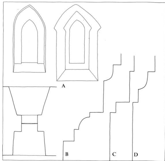
Fig. 7. A. Vindue i skibets nordside 1:40 (s. 3940), skitset af KdeFL 1993. B-D. Murede gesimser 1:10 tegnet af KdeFL efter Ole Brusendorff og Anne-Beate Nyrop 1937-38. B. Tårn, C. kor og skib, D. våbenhus. - Details of the building: A. Window in the north side of the nave, B-D. Cornices of respectively the tower, the chancel and nave and the porch.
