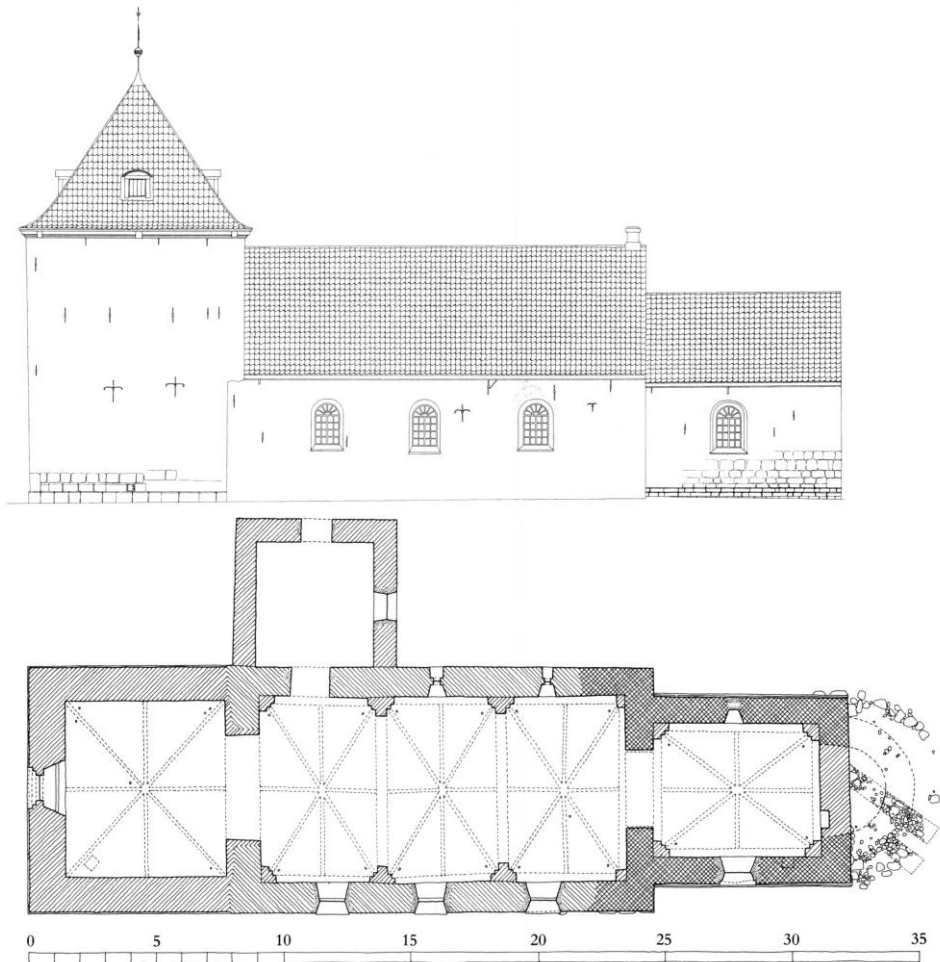
Fig. 4. Sydfacade og grundplan 1:300, henholdsvis målt og tegnet af Ole Brusendorff og Anne-Beate Nyrop 1937-38, og målt af disse, tegnet med enkelte suppleringer af KdeFL 1993. - South elevation and plan.
