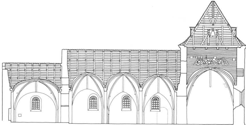
Fig. 5. Længdesnit 1:300, målt af Ole Brusendorff og Anne-Beate Nyrop 1937-38, tegnet med enkelte justeringer og tilføjelser af KdeFL 1993. - Longitudinal section.
