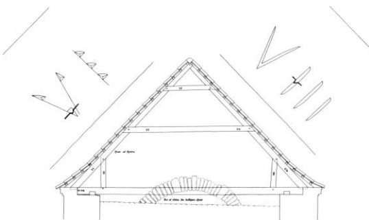
Fig. 6. Spærfag i koret 1:150 med eksempler på tømmermærker (s. 3946) samt den del af apsisbuens stik (s. 3939), som ses over hvælvet. Målt og tegnet af Ole Brusendorff og Anne-Beate Nyrop 1937-38. - Rafters of the chancel and examples of the timber marks.
