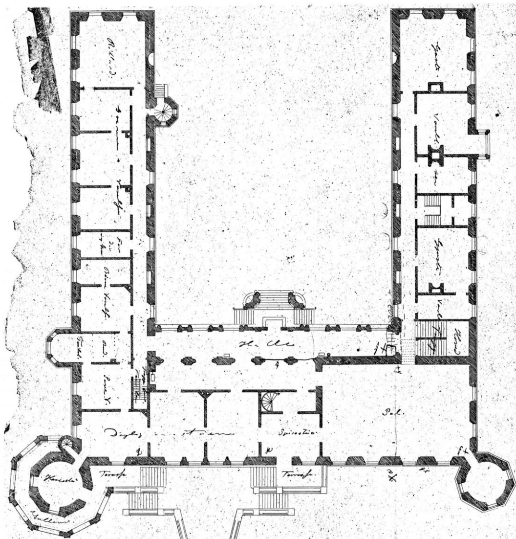
Fig. 1. Grundplan af Frijsenborgs hovedbygning før ændringer i 1860erne, sign. F. Meldahl 23. september [18]58 København. 1:400. Øst opad! Kapellet var indrettet i nordfløjens gavlværelse, der på tegningen er mærket »Billard«, NM2. - Ground-plan of the main building of Frijsenborg (before alterations in the 1860s), where a later dismantled chapel existed for a period after 1771.
