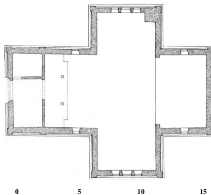
Fig. 4. Grundplan 1:300. Opmålt af Preben Hansen, Karin Stoubæk Poulsen og Anne-Mette Skifter Nielsen 1989, tegnet af KdeFL. - Ground-plan of the church, erected 1875-76.
