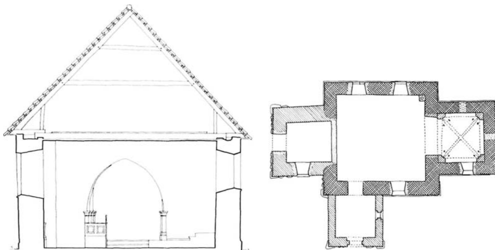
Fig. 2. Kasted. Tværsnit 1:150. Målt og tegnet af TF og KdeFL 1969. — Cross-section 1:150 . Fig. 3. Kasted. Plan 1:300. Målt af C. G. Schultz, tegnet af KdeFL 1978. — Ground-plan 1:300 .
