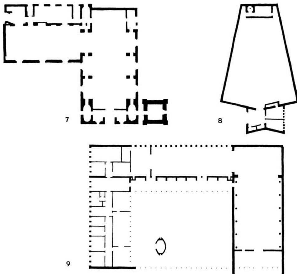
Fig. 2. Kirker i Århus kommune 1877—1966. Grundplaner 1: 600 tegnet af KdeFL. 1. Den katolske Vor Frue kirke i Ryesgade 1877—80. 2. S. Pauls kirke 1884—87 med senere tilføjelser. 3. S. Johannes kirke 1902—05. 4. Projektet »Tveje Aars« 1913. 5. S. Lukas kirke (1918—) 1921—26. 6. Christians-kirken (1937—) 1956—58. 7. S. Marcus kirke (1933—) 1934—35. 8. Møllevangskirken 1958—59. 9. Langenæskirken (1957—) 1964—66.
