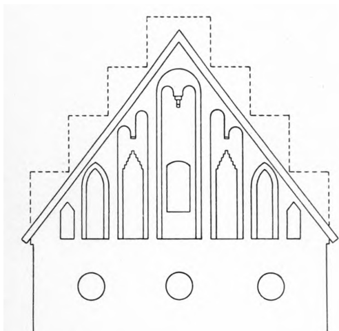
Fig. 3. Nørrejysk Blændingsgavl med antydende Kamtakker: Stigende Høj blændinger, yderst Spærstikblændinger, herefter faldede Spidsbueblændinger samt Blændinger, der afsluttes af stigende, ved en Hængestav adskilte, Rundbueblændinger og omslutter en aftrappet Blænding. Inderst Rundbueblænding omsluttende Blænding med Tvillinggrundbuer, der støttes af en kort Hængestav-Konsol. Forne den tre Cirkel- eller Bundblændinger.
