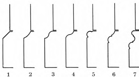
Fig. 13. Sokkelprofiler. 1. Skraakant. 2. Hul-kant. 3. Faldende Karnis. 4. Omvendt (eller forkert faldende) Karnis. 5. Rundstav. 6. Hul-kant over Rundstav. 7. Attisk.
