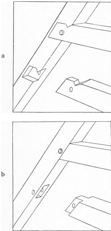
Fig. 14 a—b. Spær og Hanebaand, øverst samlet (bladet) med fornaglet Blad i Udsnit, nederst samlet (tappet) med fornaglet Tap i Taphul.
