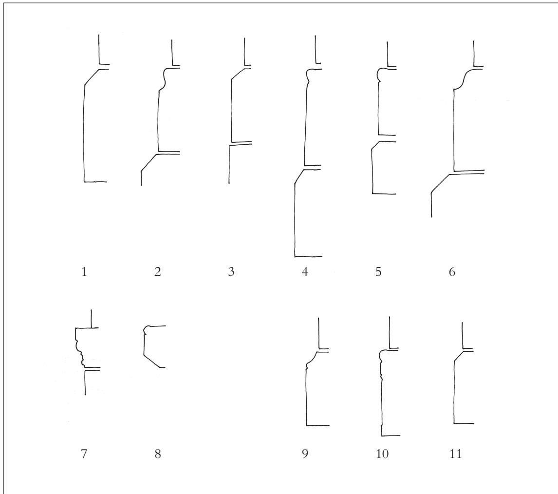
ROMANSKE BYGNINGSPROFILER i Sunds Herred, af granit. 1:10. Målt af Pia Katrine Lindholt, tegnet af Thomas Bertelsen 2018. 1. Skårup. 2. Kirkeby. 3. Stenstrup. 4. Kværndrup. 5. Bregninge. 6. Landet, sokkel. 7. Landet, korbuekrægbånd. 8. Bjerreby, korbuekrægbånd. 9. Bjerreby, sokkel på kor. 10. Bjerreby, sokkel på skib. 11. Bjerreby, sokkel på nordre korsarm. – Romanesque base profiles in granite.
