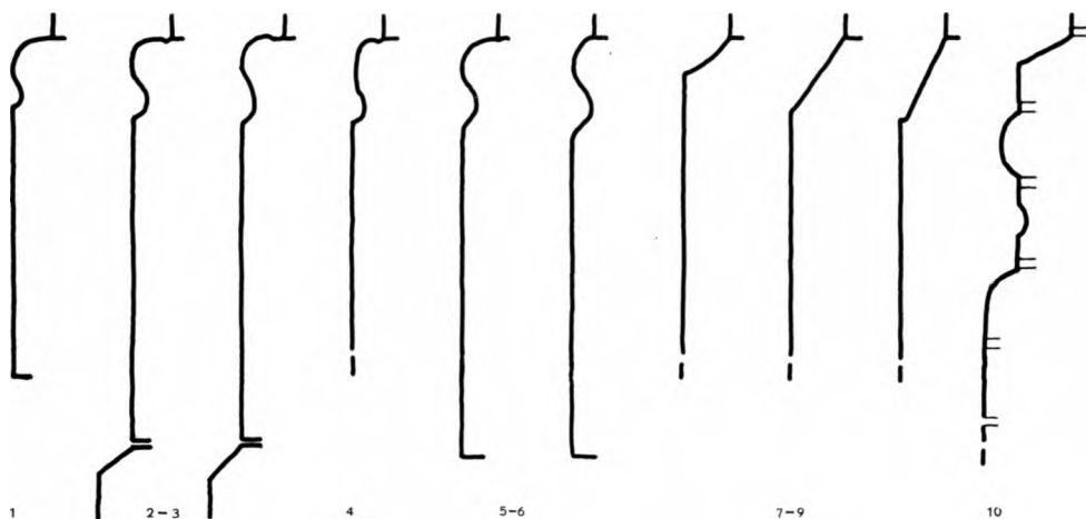
Sønderborg amt. Sokkelprofiler. 1:10. Målt af El. M.
