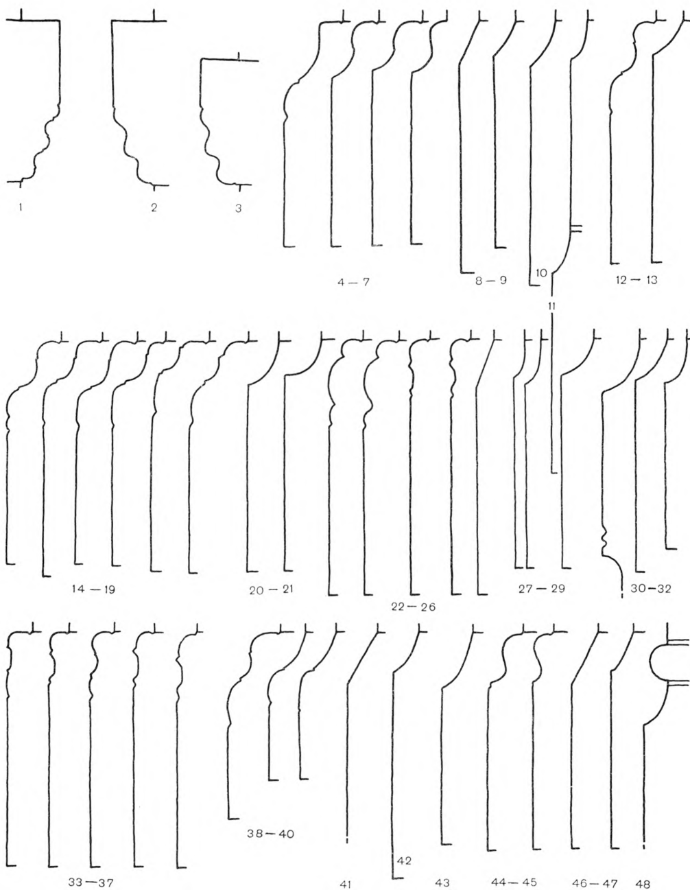
Tønder amt. Bygningsprofiler. 1:10. Målt af El. M.
