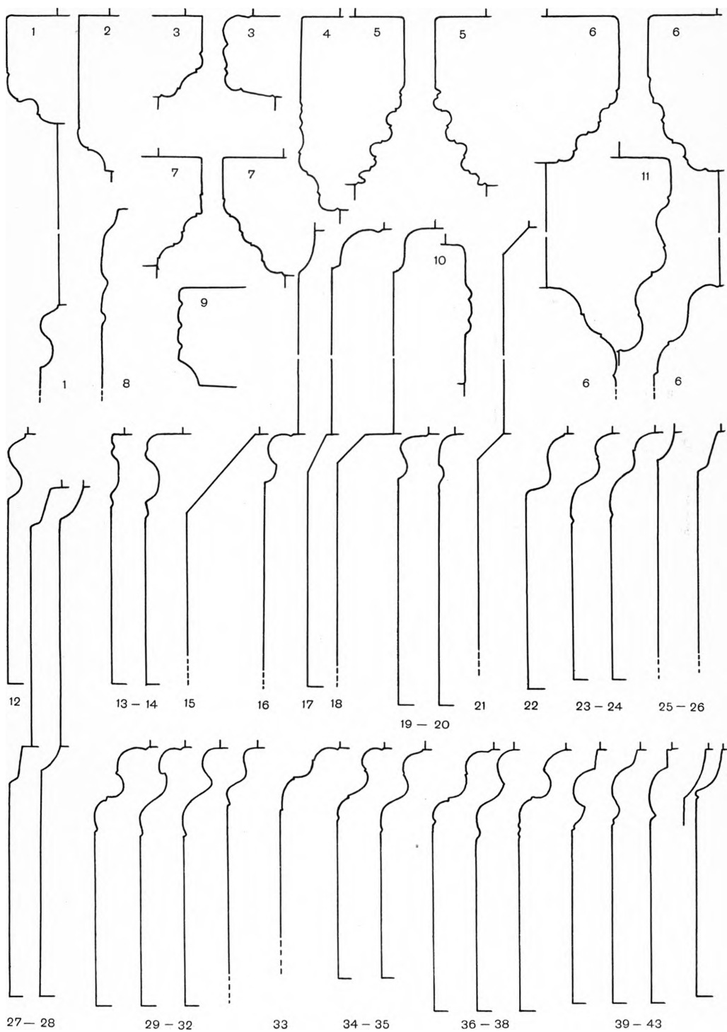
Haderslev amt. Bygningsprofiler 1:10. Målt af El. M.
