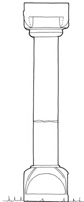
Fig. 1. Romansk søjle med base og kapitæl, antagelig fra Ribe domkirke (s. 3523). Opstillet (med basen som kapitæl) i haven ved Bramminge hovedgård. Målt af Henrik Jacobsen 1977 og tegnet af Marianne Nielsen 2003. 1:20. – Romanische Säule mit Base und Kapitell, vermutlich aus dem Dom zu Ribe.
