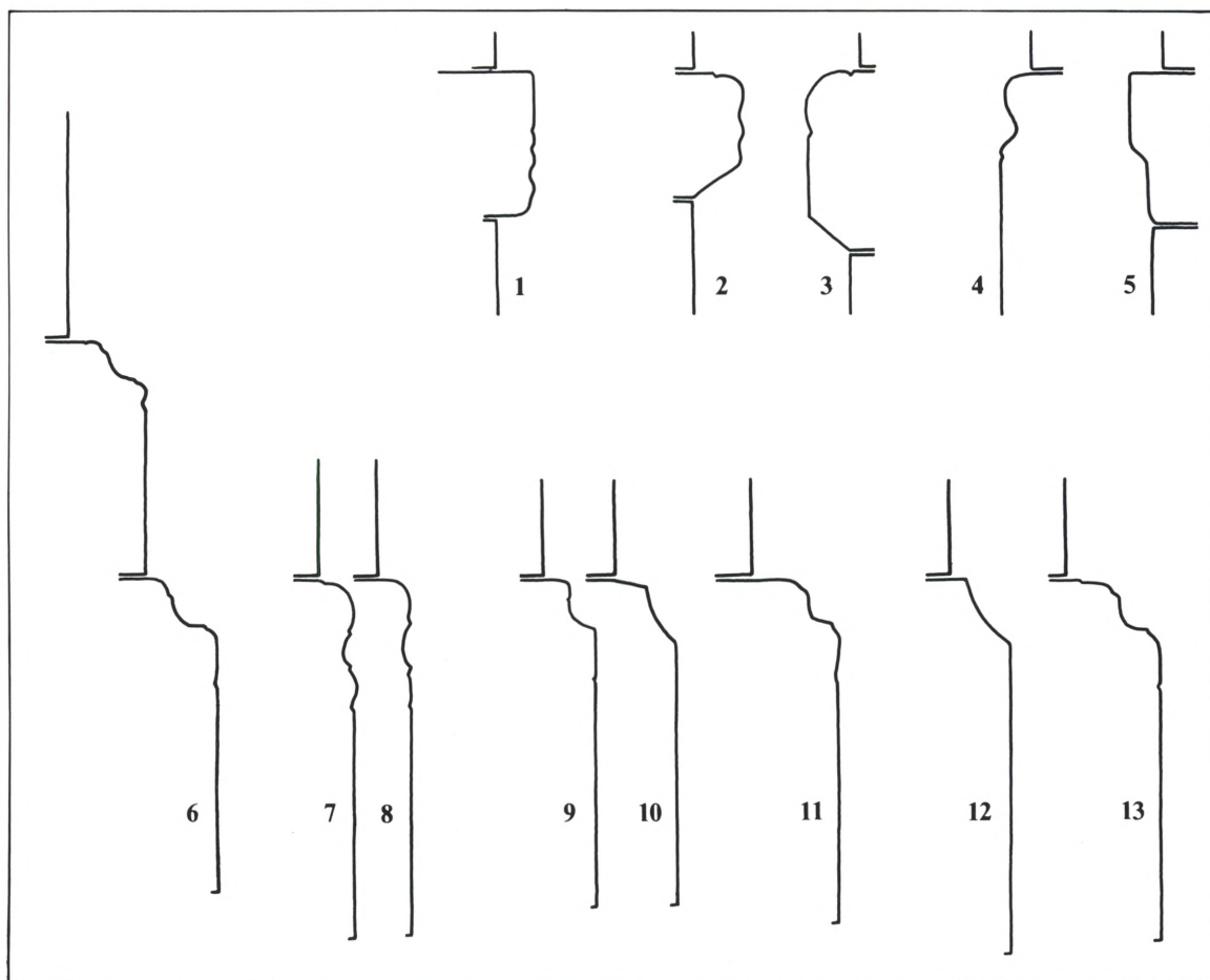
ROMANSKE BYGNINGSPROFILER i Gørding herred, af granit, 1:10. Målt af HeJ 1977 og NJP 1994, tegnet af MN 1994. Fig. 1-5: korbuekragbånd, 6-13: bygningssockler. 1. Åstrup. 2-3. Gørding. 4. Darum. 5. Jernved. 6. Gørding. 7. Darum, kor. 8. Darum, skib. 9. Bramminge, kor. 10. Bramminge, skib. 11. Vilslev. 12. Hunderup. 13. Jernved. – Romanische Gebäudeprofile aus Granit. Abb. 1-5: Kämpfer des Triumphbogens. 6-13: Sockel.
