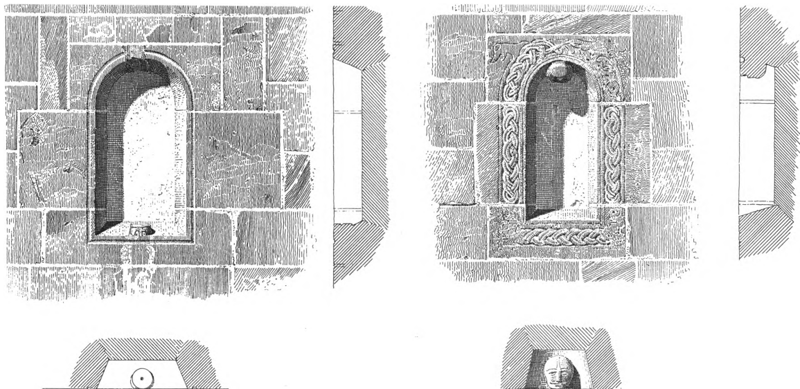
Fig. 12-13. 12. †Korets østvindue (s. 2883). 13. †Korets nordvindue (s. 2884). 1:30. Målt og tegnet af V. Koch 1892. Efter Jydske Granitkirker. - 12. Östliches Chorfenster. 13. Nordliches Chorfenster.
