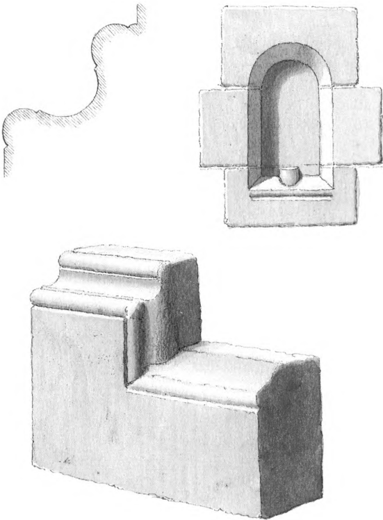
Fig. 21. Skitser af arkitekturdele i den gamle tårn kirke: sokkelprofil, korets østvindue og sydportalens vestre plint. Heinrich Hansen 1858. - Skizzen von Baufragmenten aus der alten tårn kirche: Sockelprofil, östliches Chorfenster und westliche Plinte des Südportals, 1858.
