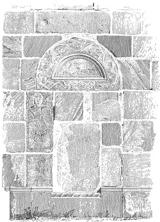
Fig. 14. Præstedør i †korets sydside (s. 2881). 1:30. Målt og tegnet af V. Koch 1892. Efter Jydske Granitkirker. - Priestertür in südlicher †Chorwand, 1892.
