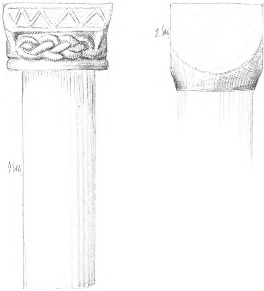
Fig. 20 a-b. *Søjlefragmenter fra tårnskibets sydportal (s. 2883), i NM. Skitse-mæssig opmåling 1:10. - *Säulenfragmente vom Südportal des tårnschiffs.
