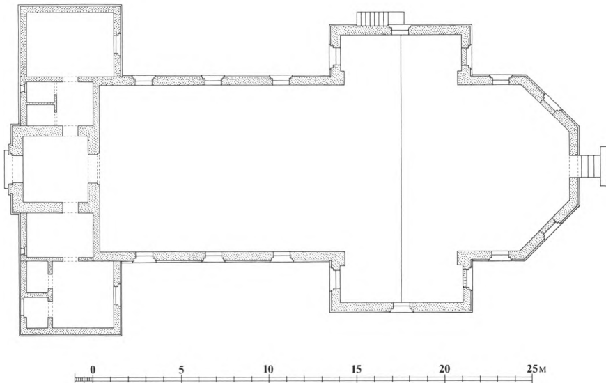
Fig. 6. Grundplan 1:300, tegnet 1994 af Marianne Nielsen med enkelte rettelser efter opmåling af Rolf Graae og Sv. Aa. Aakjær 1969. – Grundriss.
