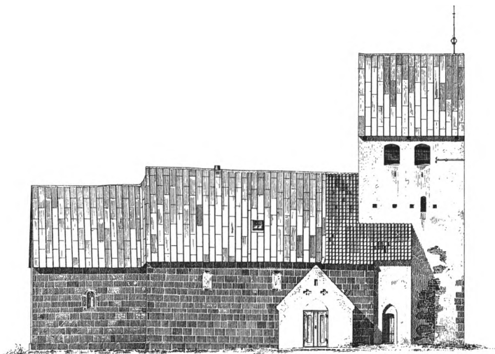
Fig. 9. Den gamle ÷kirkes nordside. 1:300. Målt og tegnet af V. Koch 1892. Efter Jydske Granitkirker . – Nordseite der alten ÷Kirche, vermessen und gezeichnet 1892.
