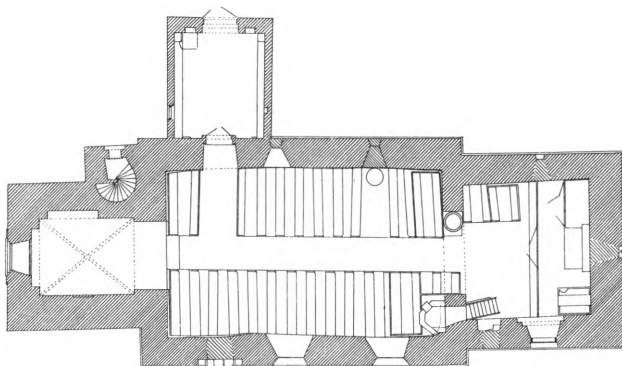
Fig. 10. Grundplan 1:300 af den gamle ÷kirke. Målt og tegnet af V. Koch 1892. Efter Jydske Granitkirker . – Grundriss der alten ÷Kirche
