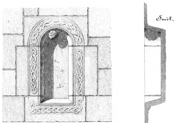
Fig. 15. †Korets nordvindue (s. 2884). 1:30. Målt og tegnet af F. Uldall 1888. – Nördliches Chorfenster.
