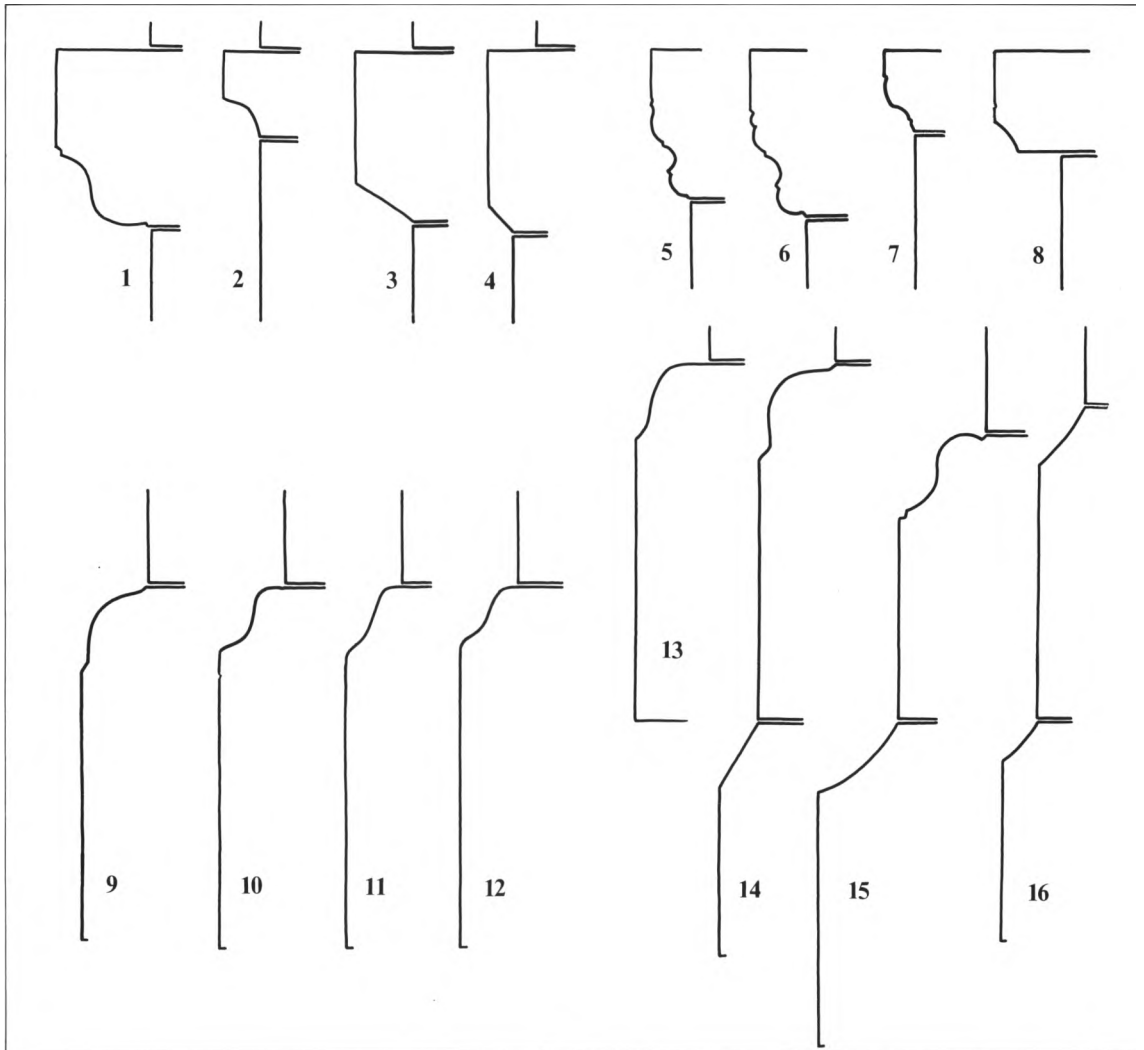
ROMANSKE BYGNINGSPROFILER i Malt herred, af granit, 1:10, målt af NJP og tegnet af MN 1993. Fig. 1-4: Kragbånd i korbue (og apsisbue). 5-8: Kragbånd i portaler. 9-16: Bygningssokler. 1. Føvling. 2. Malt. 3. Læborg, apsis. 4. Læborg, korbue. 5. Føvling, sydportal. 6. Føvling, nordportal. 7. Malt, sydportal. 8. Malt, kragbånd indsat i våbenhus. 9. Lindknud. 10. Malt, korets sydside. 11. Malt, skibets nordside. 12. Malt, tårnets sydside. 13. Brørup, nedbrudt apsis og kor samt skibets østende. 14. Brørup, skibet. 15. Føvling. 16. Læborg. – Romanische Gebäudeprofile aus Granit. Abb. 1-4: Kämpfer des Triumphbogens und Apsisbogens. 5-8: Kämpfer der Portalen. 9-16: Sockel.
