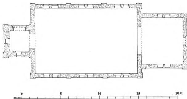
Fig. 2. Grundplan 1:300, tegnet af Marianne Nielsen 1991 efter skitse-mæssig opmåling af fimaet C. H. Hess, suppleret af Niels Jørgen Poulsen. – Grundriss .
