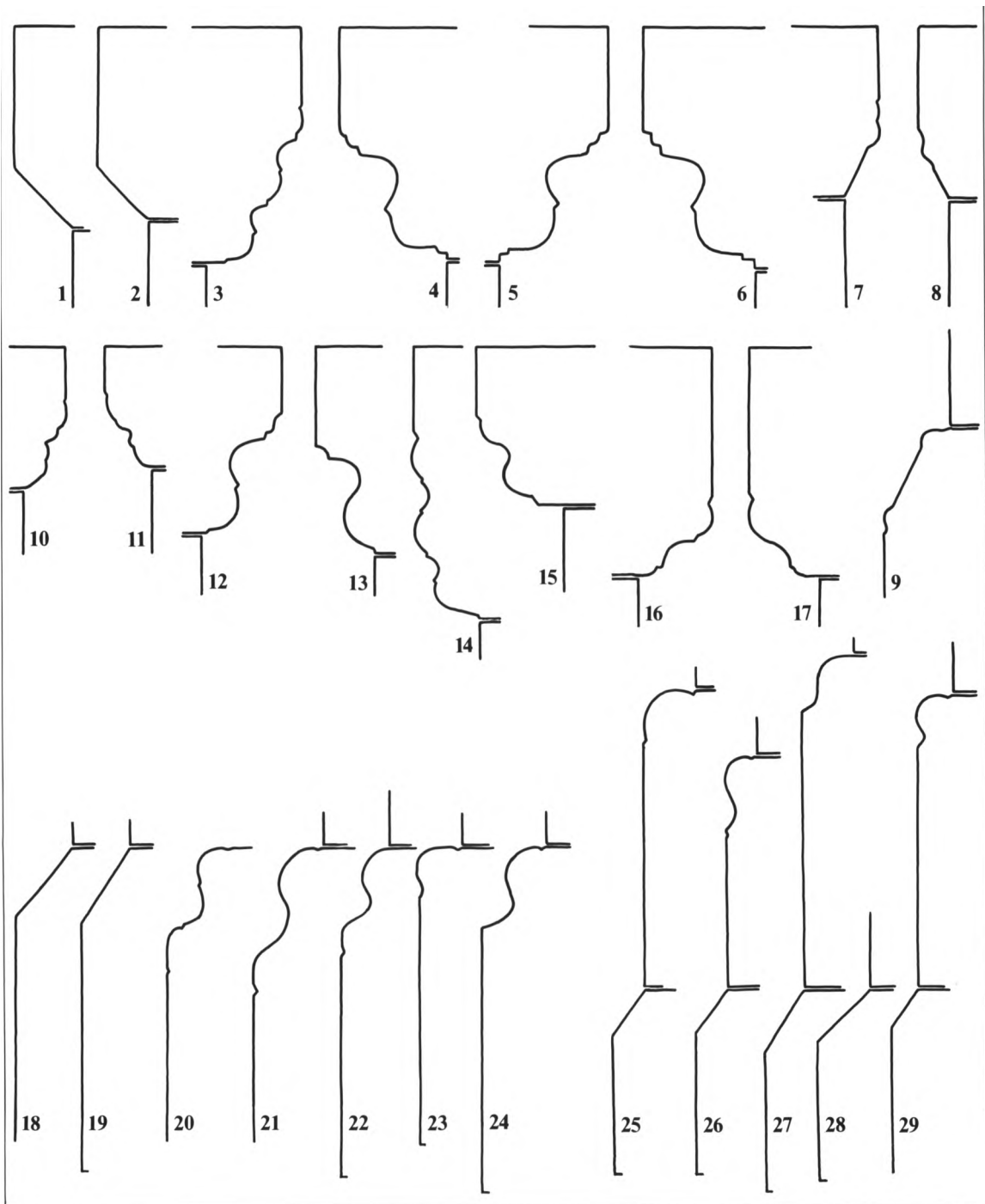
ROMANSKE BYGNINGSPROFILER i Anst herred, af granit, 1:10, målt af NJP 1991, tegnet af MN 1992. Fig. 1-13: Kragbånd i korbue (og apsisbue). 14-17: Kragbånd i portaler. 18-29: Bygningssokler. 1. Bække. 2. Hjarup. 3-4. Anst. 5-6. Anst, apsisbue. 7-8. Gesten. 9. Gesten, korbuesokkel. 10-11. Skanderup. 12-13. Vamdrup. 14. Skanderup. Norddør, østre kragbånd. 15. Vamdrup. Syddør, vestre kragbånd. 16-17. Gesten. Syddør, østre og vestre kragbånd. 18. Lejrskov. 19. Gesten. 20. Lejrskov. Kvadre i våbenhus. 21. Skanderup. 22. Hjarup, kor. 23. Hjarup, apsiskvadre. 24. Vamdrup. 25. Bække. 26. Bække, skibets sydvestre hjørne. 27. Anst, skib. 28. Anst, kor og apsis. 29. Seest. – Romanische Gebäudeprofile aus Granit. Abb. 1-13. Kämpfer und Sockel (9) des Triumphbogens und des Apsisbogens (5-6). 14-17. Kämpfer der Portalen (14. Nordportal, 15-17. Südportal). 18-29 Sockel.
