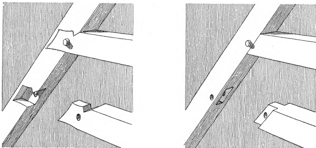
Tommerforbindelser. T. v. med foraglet Blad i Udsnit, t. h. med foraglet Tap i Taphul. Begge Forbindelser er gengivet baade i samlet og adskilt Tilstand.
