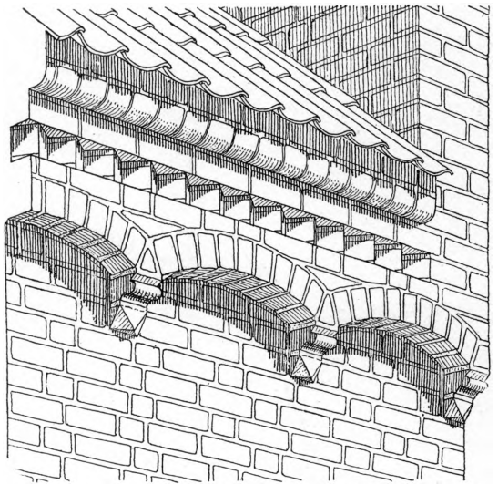
Gotisk Gesims med udkragende Fladbuer, Savskifte og afrundet Led.
