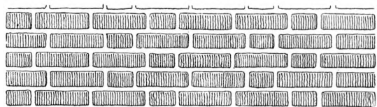
Skiftegang (Forbandt). Nederst: Munkeskifte (to Løbere, een Binder), derover: »Polsk Skifte« (een Løber, een Binder), næstøverst: Rulskifte (Bindere paa Højkant), øverst: Krydsskifte (moderne Skiftegang).
