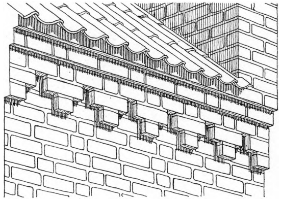
Gotisk Gesims, bloktandmuret under almindeligt retkantet Led.
