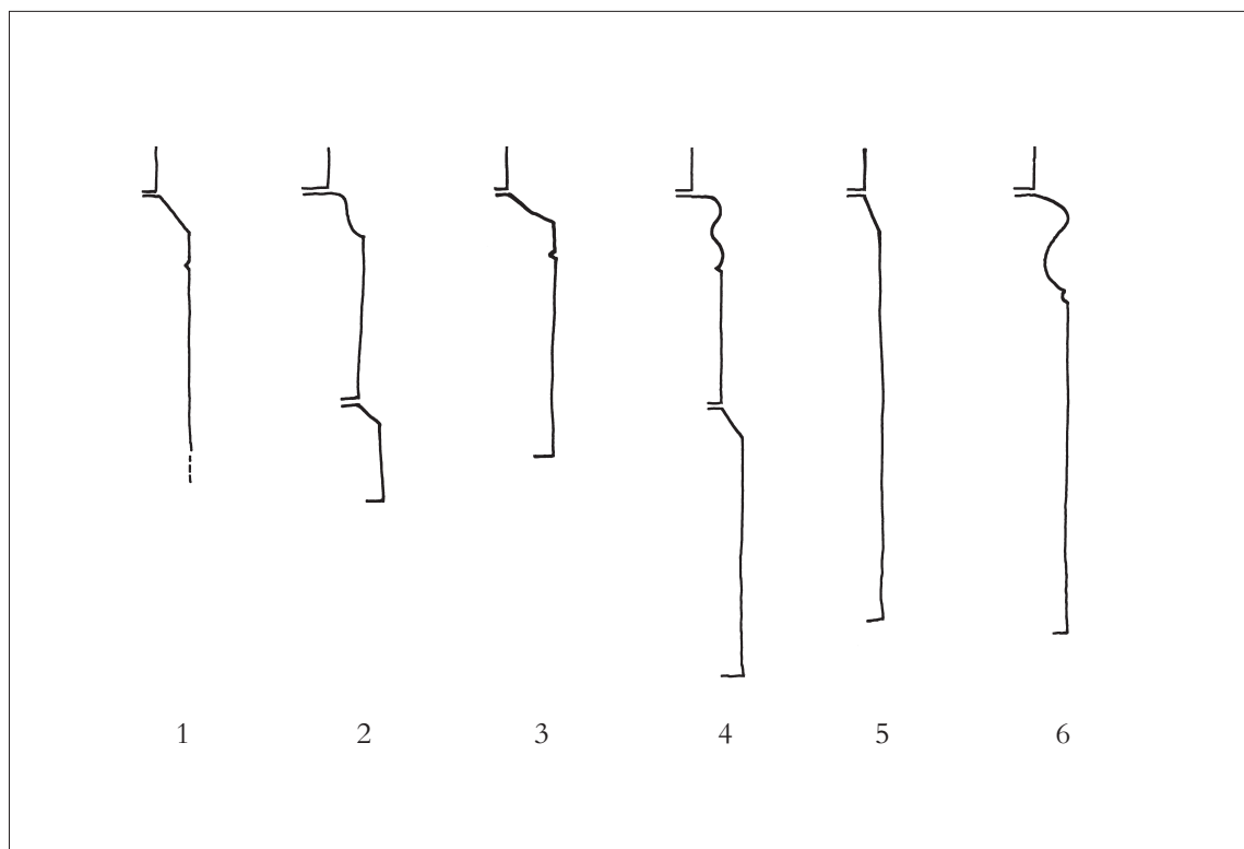
ROMANSKE BYGNINGSSOKLER i Åsum Herred, af granit, 1:10. Målt og tegnet af Kirstin Eliassen 2016. 1. Åsum. 2. Fraugde. 3. Davinde. 4. Rolfsted. 5. Sønder Nærå, tårn. 6. Nørre Lyndelse. – Romanesque base profiles in granite.
