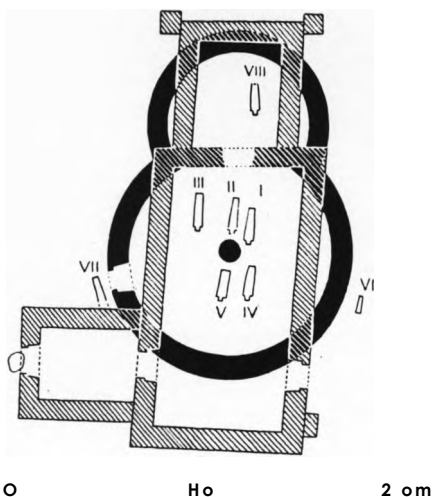
Fig. 2. Roskilde †Alle Helgens Kirke. Schematisk Fremstilling af de to Kirkers indbyrdes Forhold. C. G. S. 1944. Fra Nationalmuseets Arbejdsmark. 1950.
