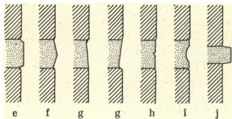
Fig. 6. Fugetyper.
