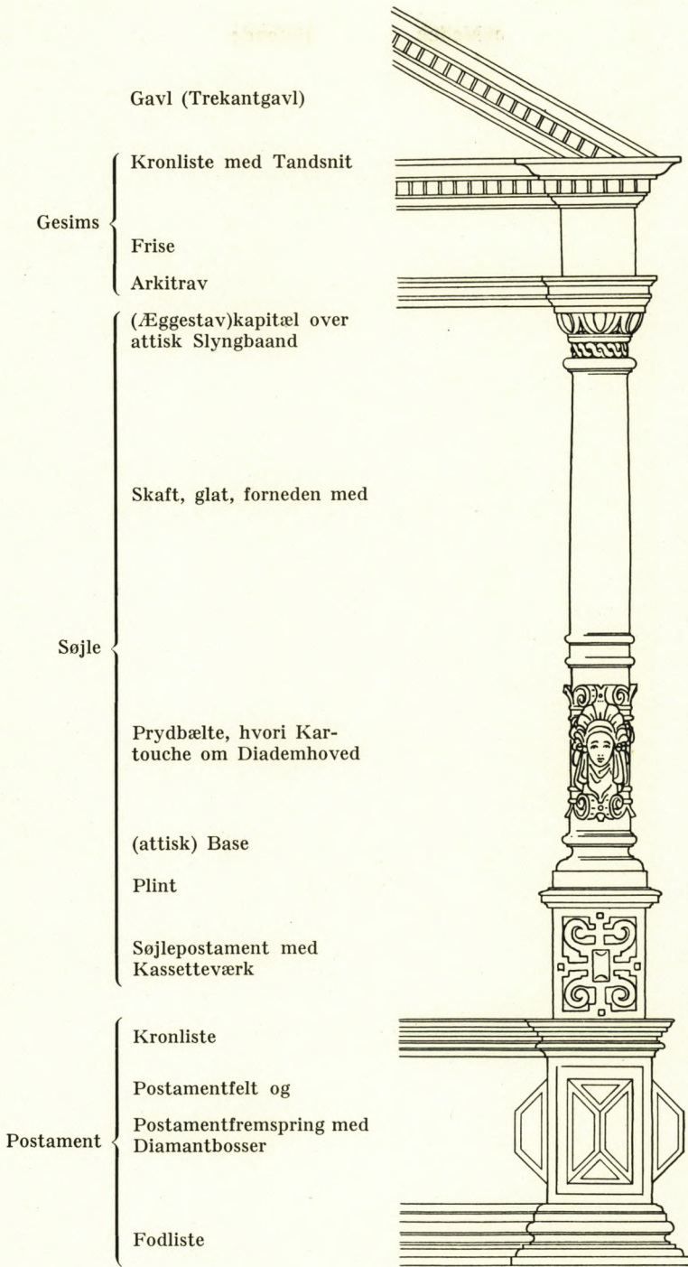
Fig. 26. Søjleskema.
