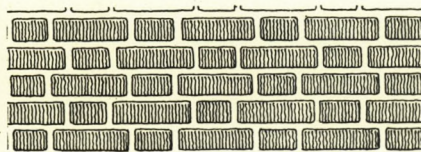
Fig. 11. Polsk Skifte.
