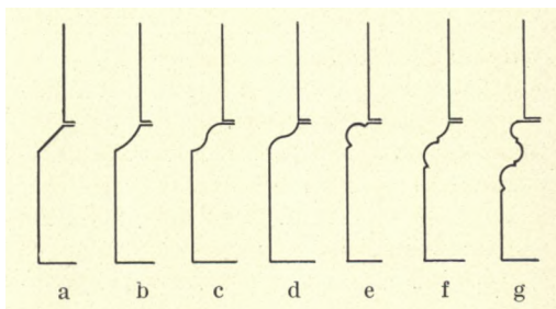
Fig. 16. Sokkelprofiler, a. Skraakant. b. Hulkant. c. Faldende Karnis. d. Omvendt (eller forkert faldende) Karnis (Klokkeprofil), e. Rundstav. f. Hulkant over Rundstav, g. Attisk.
