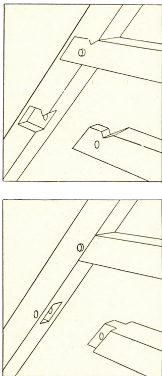
Fig. 17—18. Spær og Hanebaand, øverst samlet (bladet) med fornaglet Blad i Udsnit, nederst samlet (tappet) med fornaglet Tap i Taphul.
