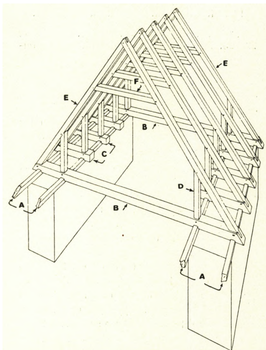
Fig. 19. Tagværk, skematisk fremstillet. A Mur-lægte (Mur-Rem). B Bjælke. C Spærsko. D Spærstiver. E Spær. F Hanebaand.
