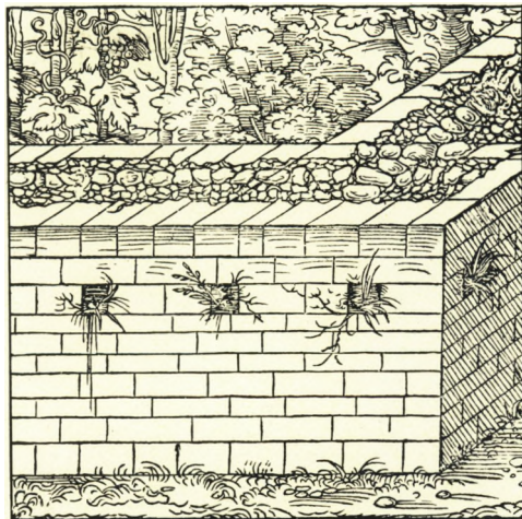
Fig. 7. Kassemur med Bomhuller. Fra Vitruvius, den tyske Udg. 1614.
