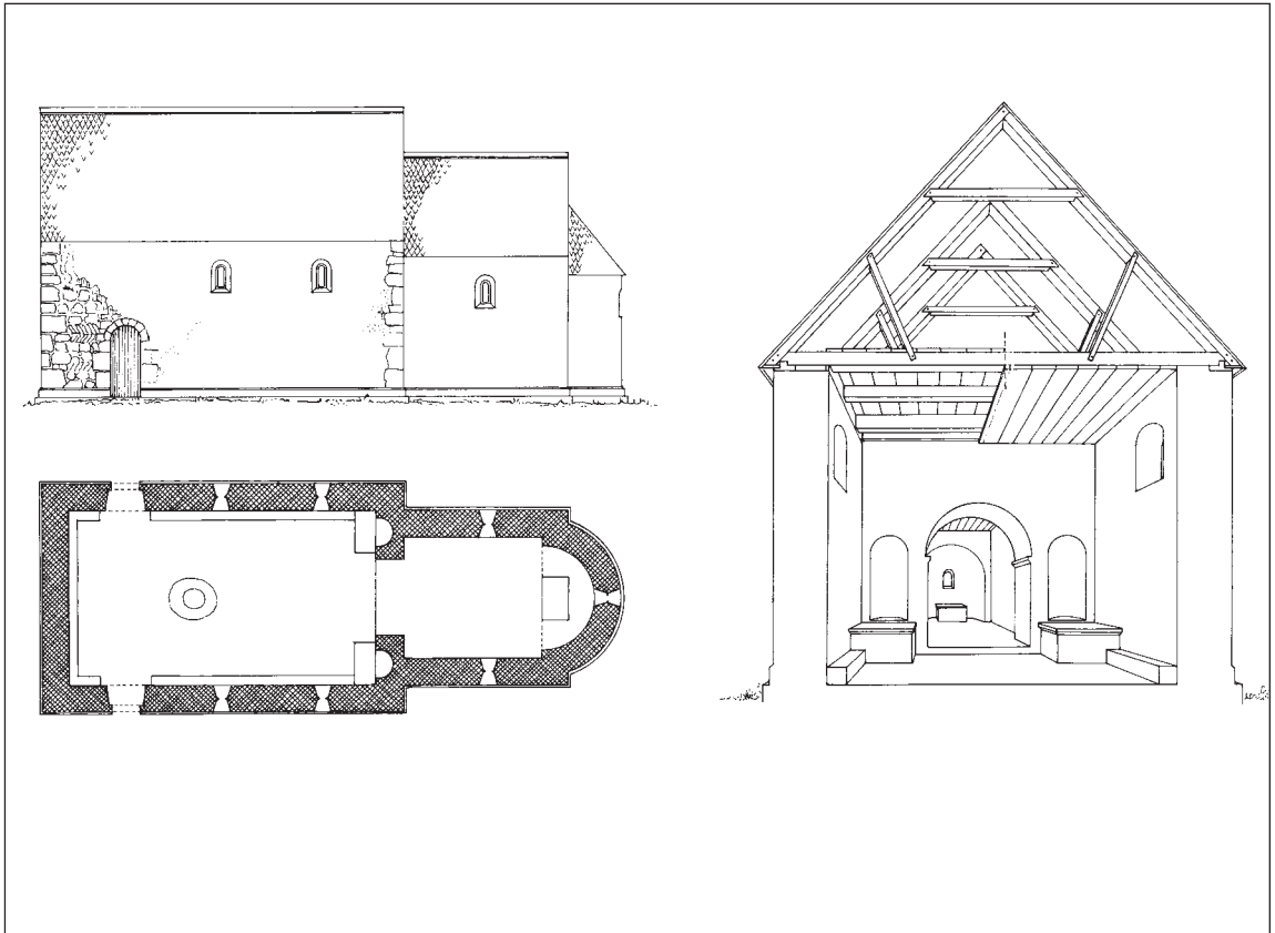
Fig. 2. Skematisk fremstilling af en romansk landsbykirke af kamp og brudsten i dens oprindelige tilstand. Hele bygningen, der består af apsis, kor og skib, hviler på sokkel med to fremspring, det underste et almindeligt, rektanglet skifte, det øverste skråkantet. Murene dækkes af puds. På skibet viser afskallet puds, at kirkens hjørner og (rundbuede) muråbninger er sat af kridt- eller frådstenskvadre af meget vekslende størrelse og format, mens murværket ellers er af rå og kløvet kamp i temmelig jævne skifter; et par steder har man udnyttet småt, flageagtigt materiale ved at stille stenene skråt, 'opus spicatum'. I lysningen af de små, højsiddende vinduer, der udvider sig tragtformet til begge sider, er der ved opførelsen indmuret egetræsrammer. Døren har rundbuet stik af kilesten. I det indre ses kirkens hovedalter stående i den med halvkuppelhvælv dækkede apsis samt, mellem kor og skib, triumfbuen, der har skråkantede kragbånd og flankeres af sidealternicher, hver med sit sidealter; ved langvæggene er murede bænke. I kor og skib er der flade lofter af planker, sømmet på undersiden af bjælkerne eller lagt ovenpå. Tagværket karakteriseres ved, at spærene, der foroven sammenholdes af hanebånd, ved hjælp af skråstivere er forstøttet ned på loftsbjælkerne (bindbjælkerne), under hvis fremspringende hoveder der som lukke i tagskægget er fastgjort sugfjæle, notet i murremmen (jf. fig. 28); de øvrige samlinger er bladede eller delvis tappede. Tagbeklædning af spån eller 'tagpander' af ældste type. Tegnet 1944 af C. G. Schultz.
