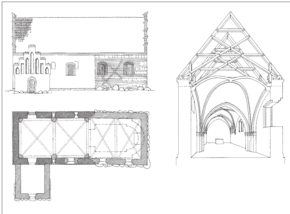
Fig. 3. Samme kirke i slutningen af middelalderen, efter flere ombygninger helt gotisk præget. I tiden o. 1350-1450 har det romanske skib fået to fag krydshvælvinger af munkesten. Som støtte for disse er der ved væggene rejst dobbeltfalsede piller, der i vederlagshøjde er afsluttet med kragbånd, hvis profil består af skråkant over rundstav, adskilt af et almindeligt skifte. Skjoldbuerne ved væggene og den tværgående gjordbue, der alle er spidsbuede og helstens brede, kantes af rundstave langs de halvtens hvælvingskapper. De halvtens ribber er uprofilerede. Af langhusets romanske vinduer er det vestre par blevet dækket af hvælvingspiller og derfor tilmurede; kun det østre par har endnu kunnet benyttes. O. 1500 er kirken blevet omdannet til en sengotisk langhuskirke, idet apsis og kor er blevet nedbrudt og skibet forlænget to fag mod øst. I stedet for sokkel har det nye bygningsafsnit en kraftig syld af store kampesten. I murværket, der står blankt, er en del romanske kridt- og frådstenskvadre blevet genanvendt og ses uregelmæssigt fordelt i bæltet, men ellers er materialet munkesten i munkeskifte, de mørkbrændte sten formuret som bindere, der enkelte steder danner en slags rudemønster. I syd ses i hvert af de to fag et stort falsat, fladbuet vindue; et tilsvarende har samtidig fortrængt det sydøstligste af skibets romanske vinduer. I det indre er de samtidige hvælv indbygget i væggene, hvorfor hvælvingspiller og særlige skjoldbuer mangler. Kun i sammenstødet med det østligste af de ældre hvælv i skibet har det været nødvendigt at opføre en ekstra gjordbue, hvilende på spinkle vægfremspring. Hvælvingerne er i øvrigt af samme type som skibets, dog mangler der rundstave langs kappekanterne. Op ad østvæggen ses kirkens hovedalter. Ved samme lejlighed er det romanske skibs mure blevet forhøjet, og hele bygningen har fået muret gesims, bestående af to udkragede skifter, samt nyt tagværk og nye gavle. Tagværket, der har to lag hanebånd, er af krydsbåndstype. Hvert krydsbånd er fornedet bladet til den korte, vandrette spærsko, krydser den på denne rejste spærstiver samt, højere oppe, det underste hanebånd og er med sin anden ende bladet fast til det modsatte spær. Gavlene har kamtakker, afdækket med munketeg (munke og nonner); hele taget er hængt med det samme materiale. Foran syddøren er der rejst et våbenhus. Døren, der er falsat, er rundbuet med spidsbuet spejl. Gavlens dekoration består af syv højblændinger med varierende afdækninger – afrappet, vandret, spærstikformet og spidsbuet. De hertil svarende syv kamtakker afsluttes foroven med svage, vandrette udkragninger, 'bryn', og er hængt med munketeg. I denne sengotiske langhuskirke har der ikke været noget egentligt arkitektonisk markeret skel mellem kor og skib som i den ældre, romanske. I stedet har det som kor tjenende østligste fag været adskilt fra resten af kirken ved et trægitter (ikke vist på tegningen), foran hvilket eventuelle sidealtre har været anbragt. Tegnet 1944 af C. G. Schultz.
