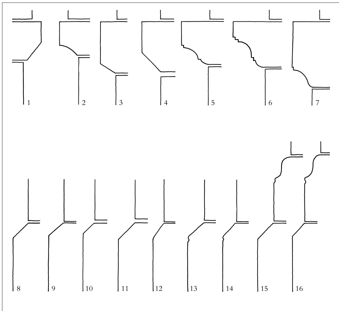
ROMANSKE BYGNINGSPROFILER i Vandfuld Herred, af granit, 1:10. Målt af Peter Duun 2009-10 og Hugo Johannsen 2011, tegnet af Merete Rude 2011. Fig. 1-7: Korbuekrægbånd. 8-16: Bygningssokler. 1. Engbjerg (nord). 2. Engbjerg (syd). 3. Dybe. 4. Ferring. 5. Trans. 6. Hove. 7. Hygum. 8. Ramme. 9. Fjaltring. 10. Trans. 11. Ferring. 12. Engbjerg. 13. Dybe. 14. Hygum. 15. Hove. 16. Vandborg. – Romanische Gebäudeprofile aus Granit in der Härde von Vandfuld. Abb. 1-7. Kämpfer des Triumphbogens. Abb. 8-16. Sockel.
