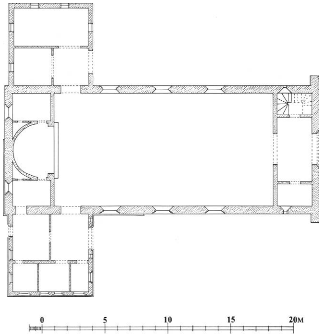
Fig. 5. Kapel på Vestre kirkegård. Plan 1:300. Efter opmåling af Søren Jensen 1993, tegnet af MN 2000. - Leichenhalle auf dem Westfriedhof, Grundriss.
