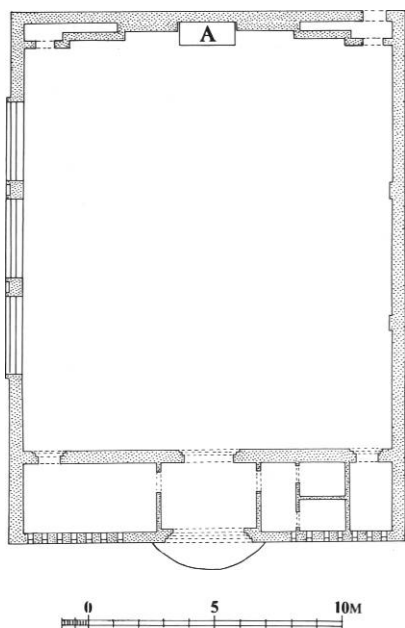
Fig. 3. Plan 1:300. Efter forslag af Niels Bygum Clausen 1950, suppleret af NJP og tegnet af MN 2000. - Grundriss.
