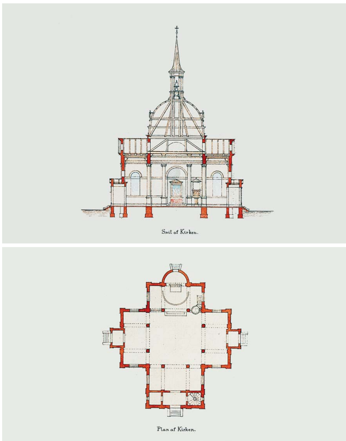
Fig. 1a-b. Vilhelm Petersens indledende forslag til en kirke ved Statshospitalet (s. 2411). Snit og plan (uden mål). Foto Arnold Mikkelsen 2010. – Vilhelm Petersen's initial proposal for a church at the State Hospital.
