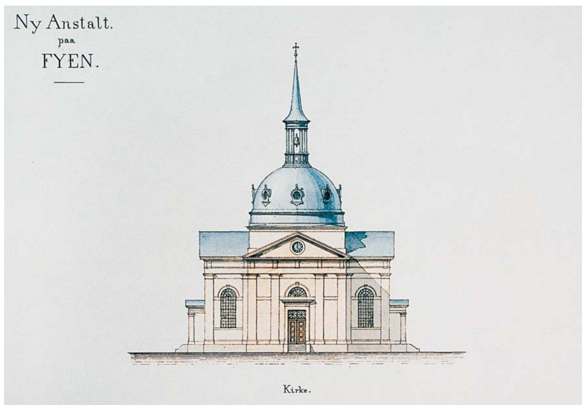
Fig. 1c. Vilhelm Petersens indledende forslag til en kirke ved Statshospitalet (s. 2411). Opstalt (uden mål). Foto Arnold Mikkelsen 2010. – Vilhelm Petersen's initial proposal for a church at the State Hospital.
