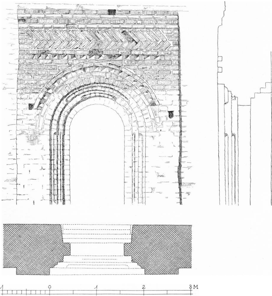
Fig. 3. Vaalse. Sydportal. 1:50. Målt af Aa. Rl. 1940 (s. 1203).
