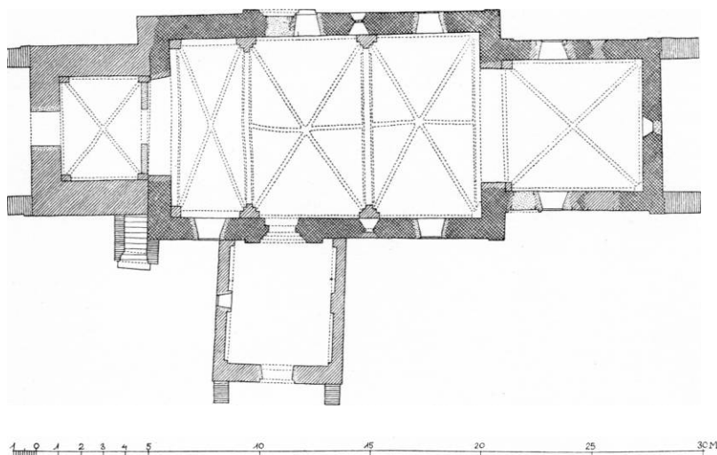
Fig. 2. Vaalse. Plan. 1:300. Målt af Aa. Rl. 1940.
