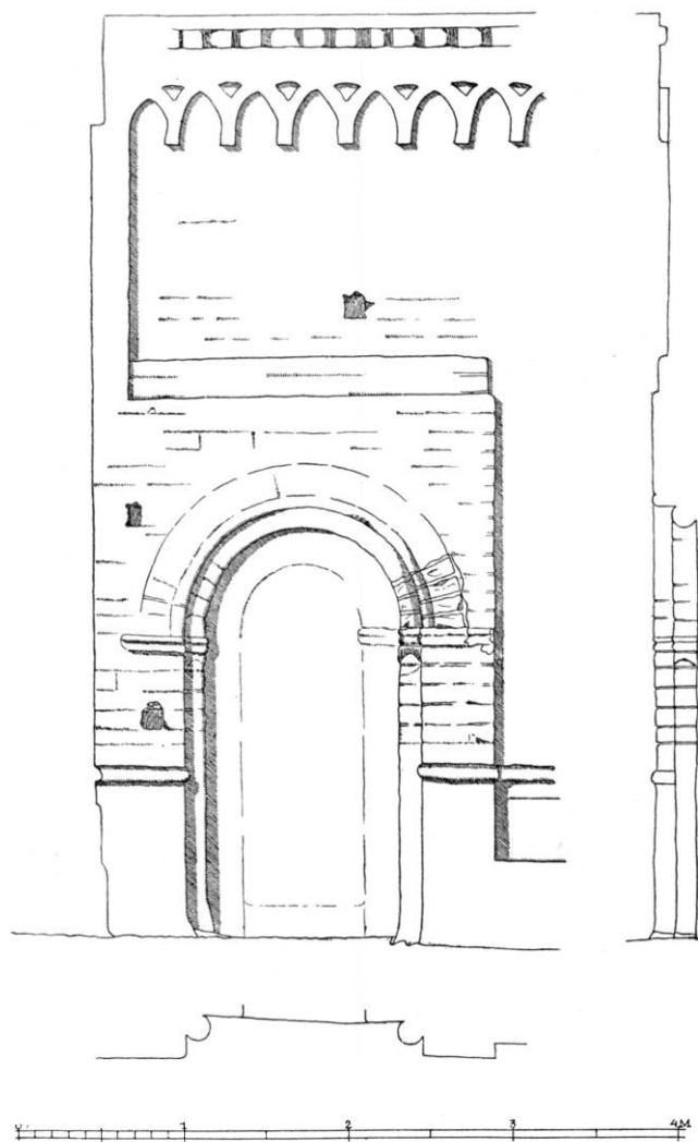
Fig. 4. Øster-Ulslev. Præstedør i korets sydside. 1:50. Målt af F. B. Jørgensen 1944 (s. 1062).
