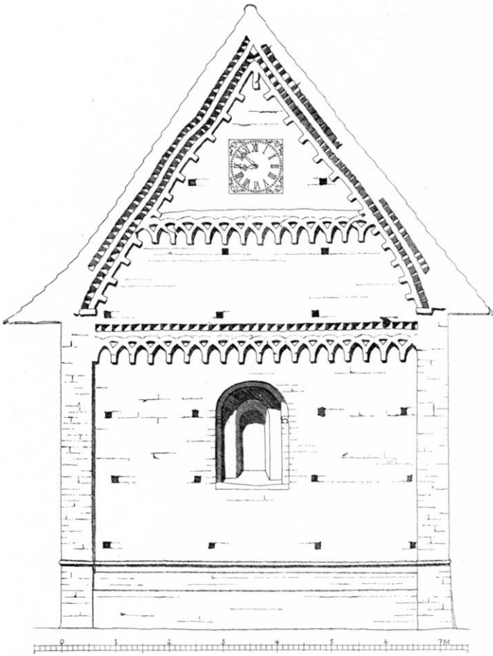
Fig. 3. Øster-Ulslev. Korets ostgavl. 1:100. Målt af Frithiof Lange 1944 (s. 1062).
