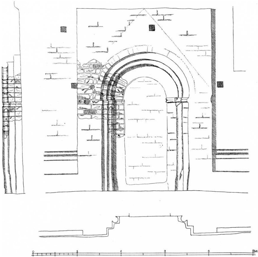
Fig. 5. Øster-Ulslev. Nordportal. 1:50. Målt af B.F.Lorentzen 1944 (s. 1063).
