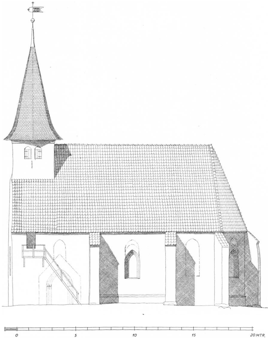
Fig. 3. Engestofte. Sydfaçade. 1:200. Målt af Tove Bojesen 1942.
