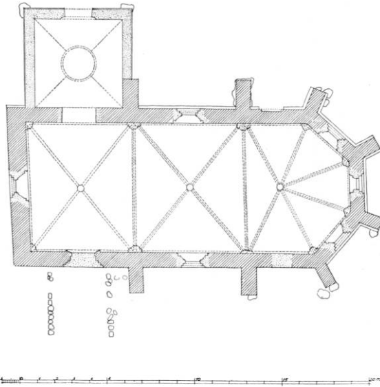
Fig. 2. Engestofte. Plan. 1:300. Målt af Olav Schiorring 1942.
