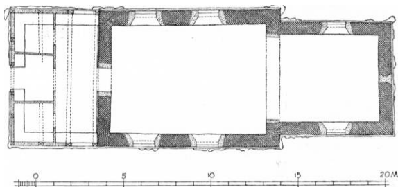
Fig. 2. Skørringe. Plan. 1:300. Målt af Elna Møller 1948.
