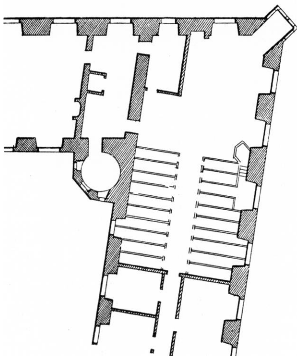
Fig. 3. †Nykøbing slotskirke. Plan af den reformerte kirke. 1:300. Udsnit af Thuras plan.
