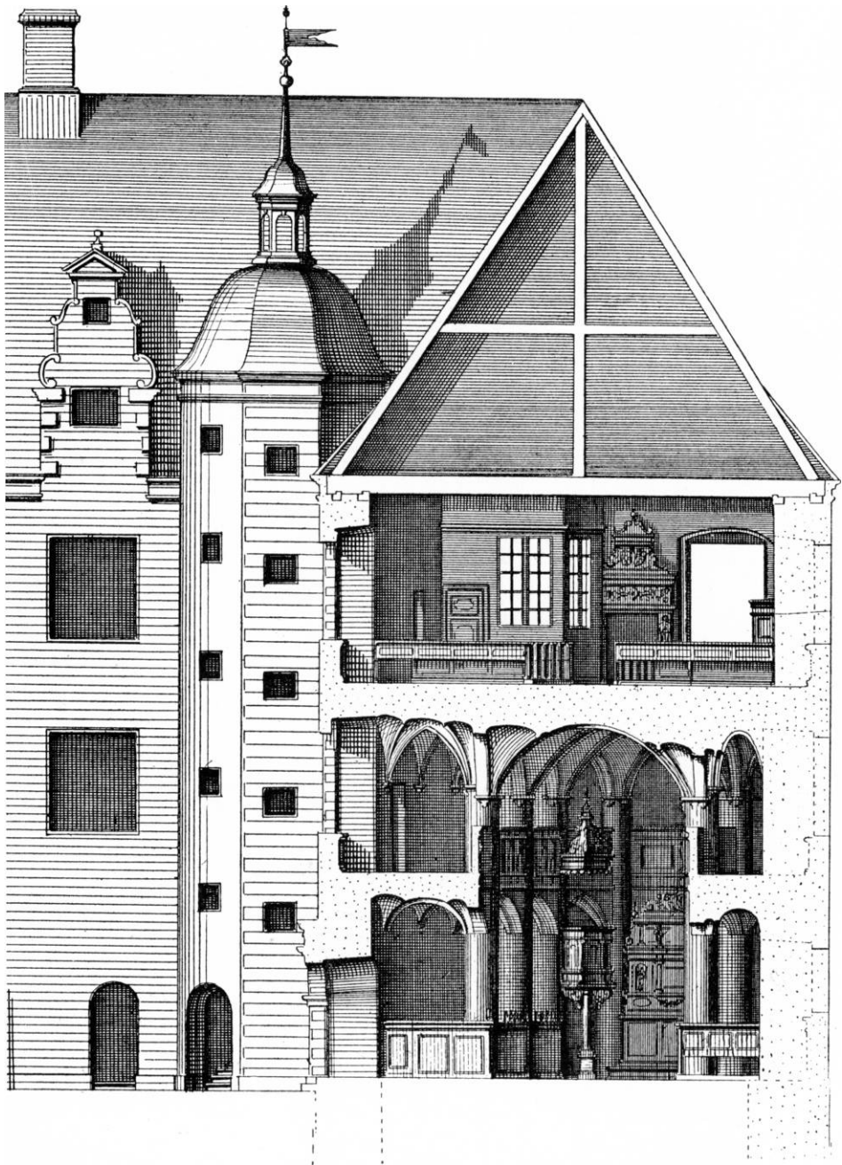
Fig. 2. †Nykøbing slotskirke. Snit af østfløjen. 1:150. I de to nederste stokværk renaissancekirken, i det øverste den reformerte kirke. Efter Thura.
