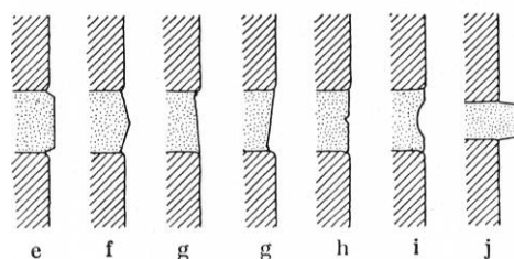
Fig. 5. Fugetyper.
