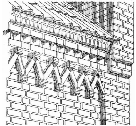
Fig. 8. Spærfrise.
