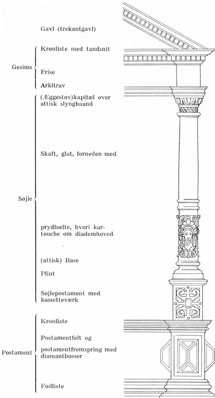
Fig. 23. Søjleskema.
