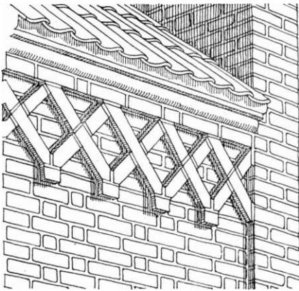
Fig. 7. Rudefrise.
