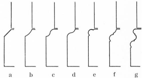
Fig. 19. Sokkelprofiler, a. Skraakant. b. Hulkant. c. Faldende karnis. d. Omvendt (eller forkert faldende) karnis (klokkeprofil). e. Rundstav. f. Hulkant over rundstav. g. Attisk.
