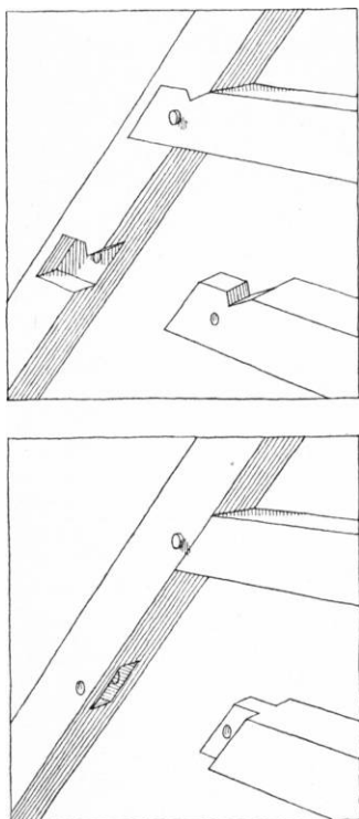
Fig. 20—21. Spær og hanebånd, øverst samlet (bladet) med fornaglet blad i udsnit, nederst samlet (tappet) med fornaglet tap i taphul.
