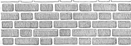
Fig. 14. Polsk (vendisk) skifte.
