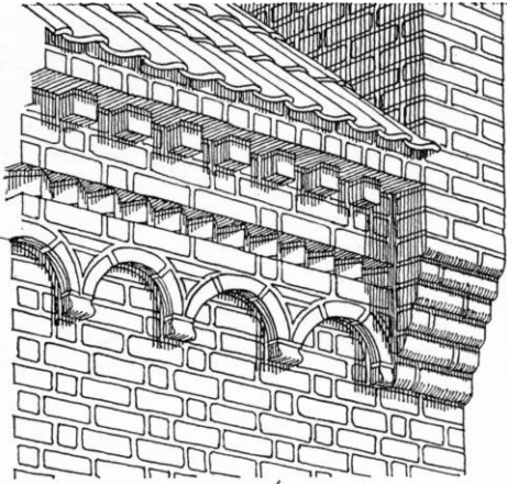
Fig. 9. Enkelt rundbuefrise.
