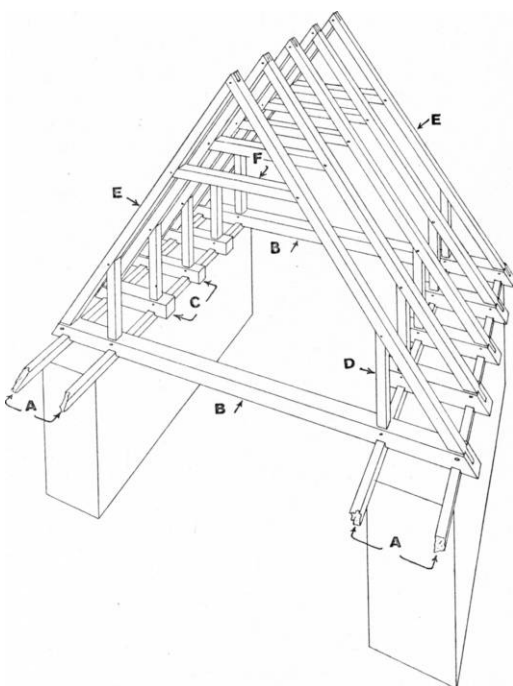
Fig. 22. Tagværk, skematisk fremstillet. A mur-lægte (mur-rem). B bjælke. C spærsko. D spærstiver. E spær. F hanebånd.
