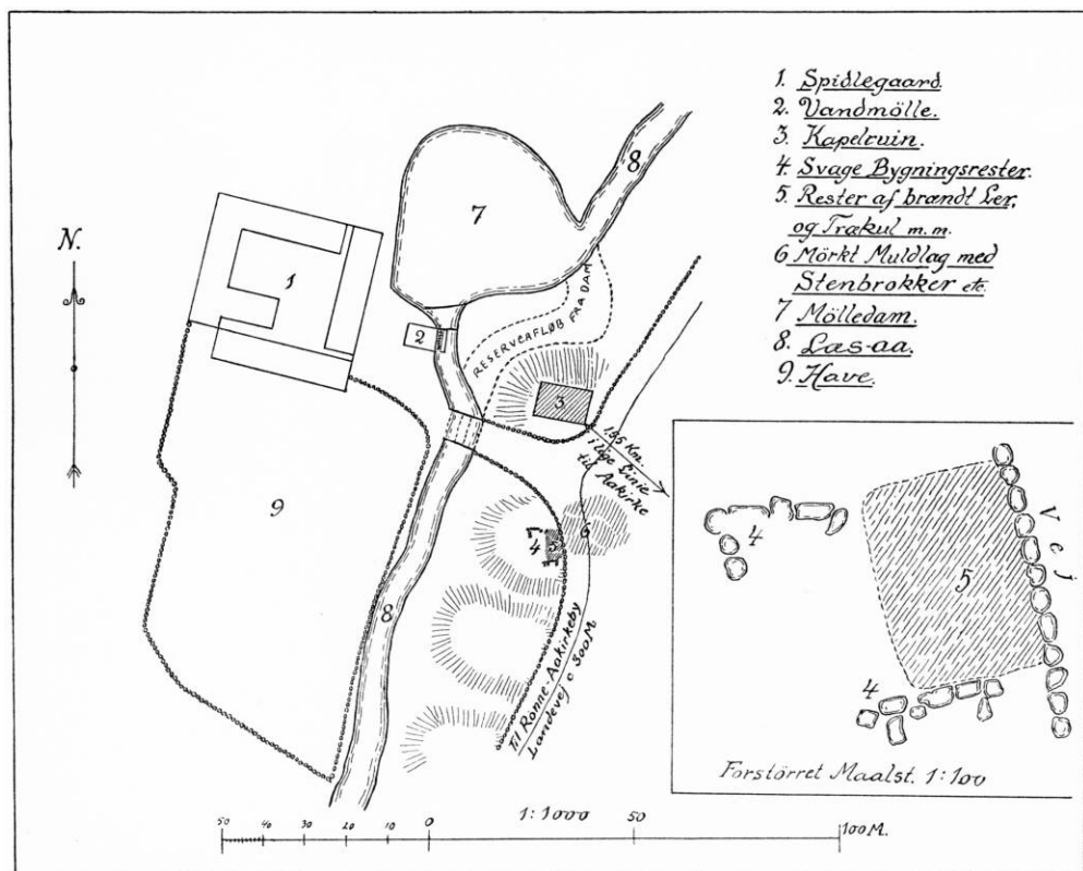
Fig. 1. S. Jørgens-Kapellet ved Spidlegård. Situationsplan, 1:2000 (indsatsen 1:200). Efter tegning af arkitekt K. S. L. Thorsen 1918.
