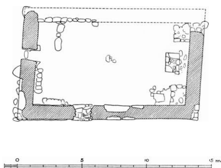
Fig. 2. S. Jørgens-Kapellet ved Spidlegård. Grundplan, 1:300, målt af K. S. L. Thorsen 1918. Tegnet af Tove Bojesen 1952.
