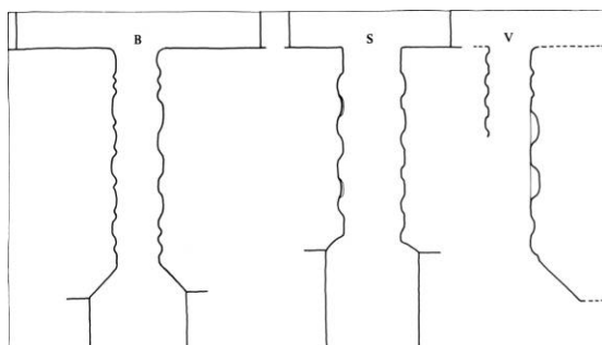
Romanske bygningsprofiler i Hjelslev herred 1:10, målt og tegnet af KdeFL. B: Blegind kirke: Sydportalens kragbånd. Et løstliggende kragbånd, der nu befinder sig på Blegindgård, er ikke medtaget. S: Stilling kirke: Nordportalens kragbånd (s. 2946). V: Vitved kirke: Kragbånd (?), indmurede i tårnunderdelen (s. 3024). Det til højre antagelig fra den oprindelige triumfbue. - Romanesque building mouldings in the district of Hjelslev.
