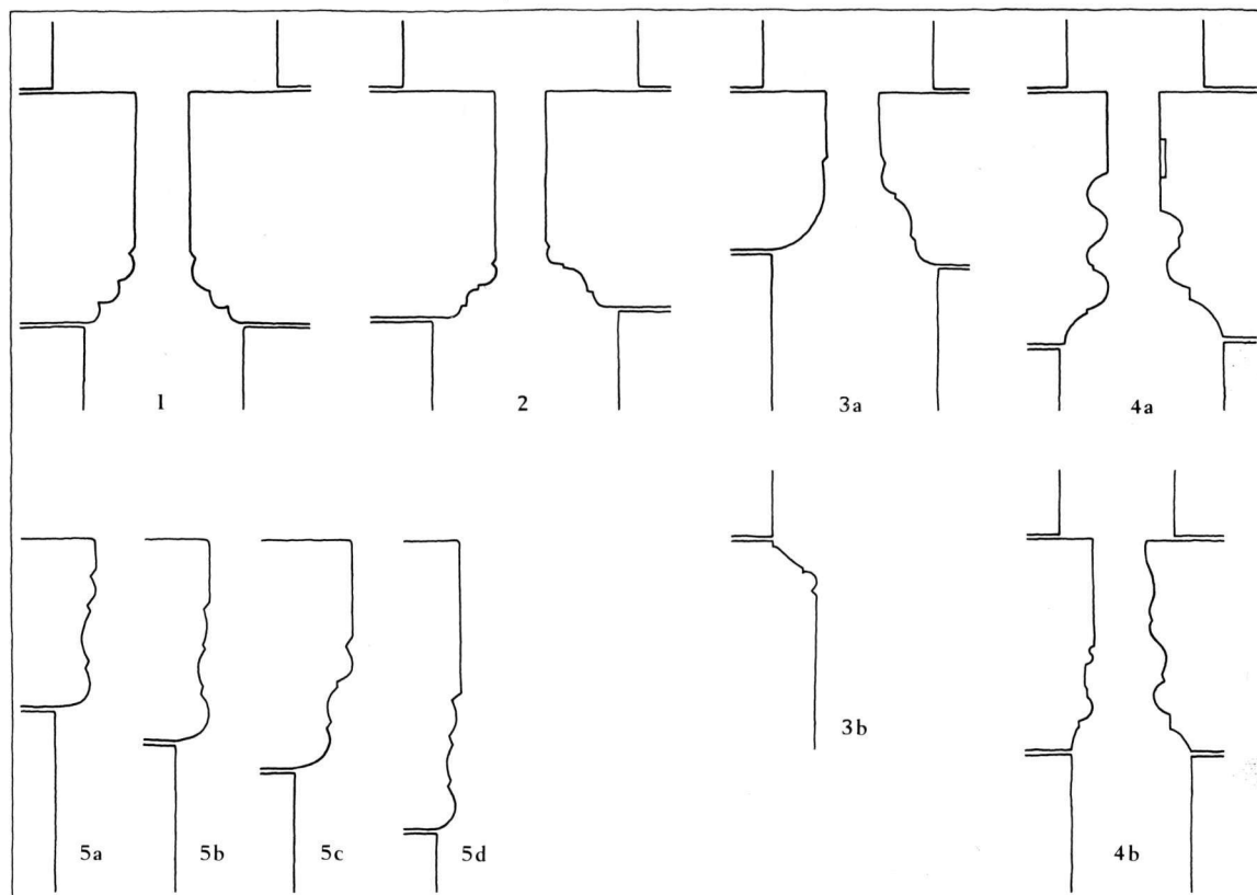
Romanske bygningsprofiler i V. Lisbjerg hrd., med Lading (Sabro hrd.), 1:10, målt af KdeFl og NJP, tegnet af Flemming Beyer. Øverst korbuekragsten: 1. Elev. 2. Lading. 3a. Trige. 4a. Elsted. 5a-d. Spørring: a-b. Sydportalens kragsten. c. Korbuekragsten, nu i tårnets sokkel. d. Apsidens gesims. 3b. Trige, sokkel. 4b. Elsted, sydportalens kragsten. - Romanesque building stones in the district of V. Lisbjerg, including Lading.
