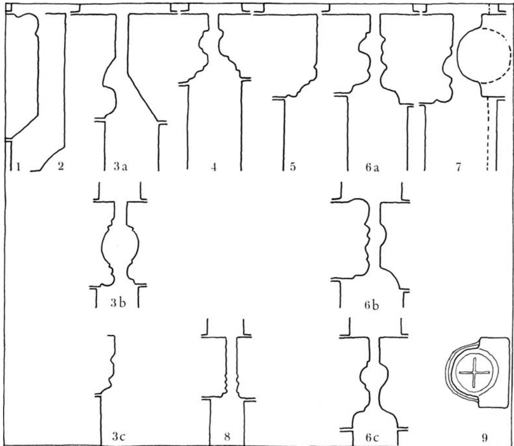
Romaneske, profilerede bygningssten i Hasle herred, inklusiv Skejby, 1:10, målt af KdeFL. Øverste række: Korbuekragssten. Mellemste række: Kragsten i sydportaler. Nederste række: Kragsten i nordportaler. 1. Hasle. 2. Lyngby (løsliggende sten). 3a—c. Tilst. 4. Brabrand. 5. Skejby. 6a—c. Vejlbj. 7. Åby. 8. Årslev. 9. Kragsten i Den gamle By. Inv. nr. 656:55 (p. 1360). — Romanesque moulded building stones in the district of Hasle, including Skejby, 1:10. Top row: corbels in chancel arch. Middle row: corbels in south portals. Bottom row: corbels in north portals.
