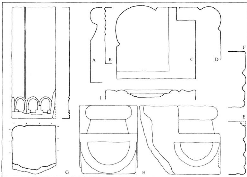
Fig. 10. Ikke lokaliserede, profilerede bygningsblokke af granit, 1:10. Stenene, der nu befinder sig i Den gamle By, stammer antagelig fra Århusområdet (p. 1359f). Målt og tegnet af KdeFL 1974. — Granite profiled building stones 1:10 of unknown siting. The blocks, now in the museum »Den gamle By«, originate presumably from the Århus area.
